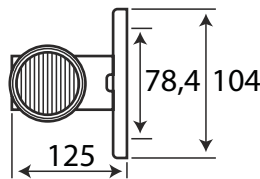
▪ Universal LED Begrenzungsleuchte
