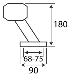
▪ Universal LED Begrenzungsleuchte
