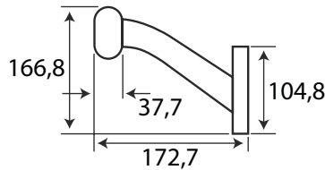
▪ Universal LED Begrenzungsleuchte
