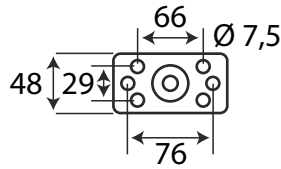
▪ Universal LED Begrenzungsleuchte
