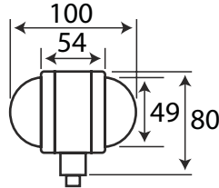
▪ Universal Begrenzungsleuchte
