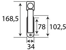
▪ Universal LED Begrenzungsleuchte
