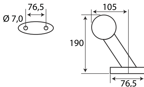
▪ Universal LED Begrenzungsleuchte
