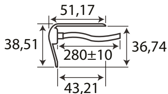
▪ Universal Innenbeleuchtung
