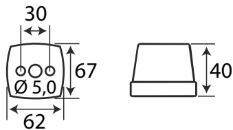
▪ Universal Begrenzungsleuchte
