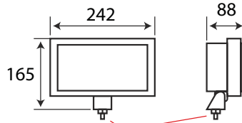
Befestigungsschraube M10 mounting screw M10
